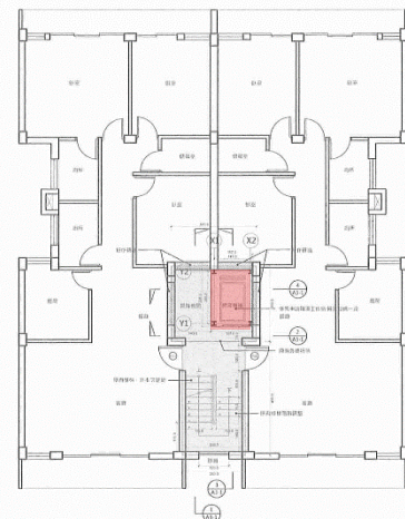
2 A2-1 貳層平面圖 Scale 1/100
