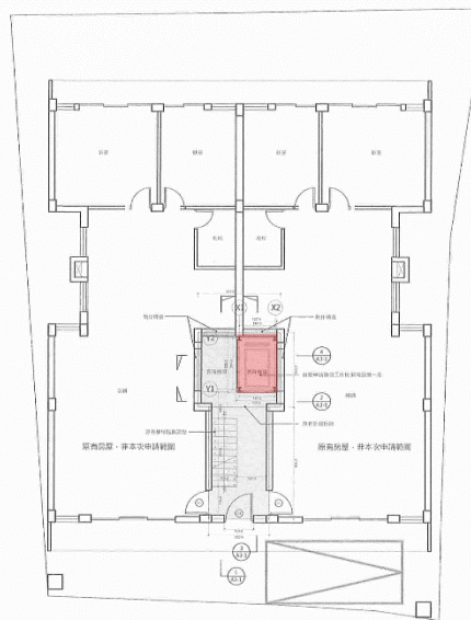
1 A2-1 壹層平面圖 Scale 1/100
